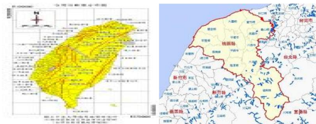
圖 2-2-1、活動斷層圖
